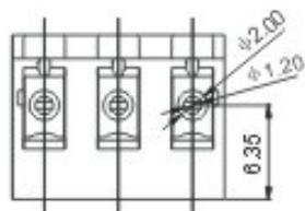
A 向视图
