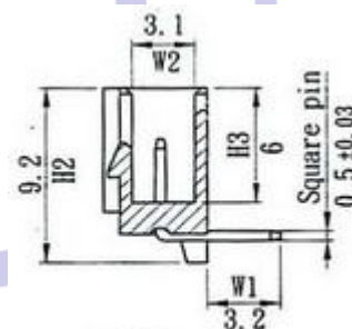
A-A Section
